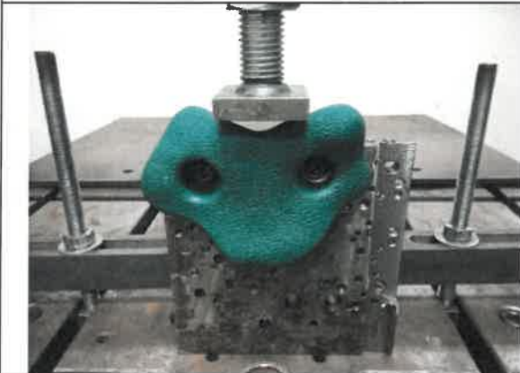
Photo C : Test setup
